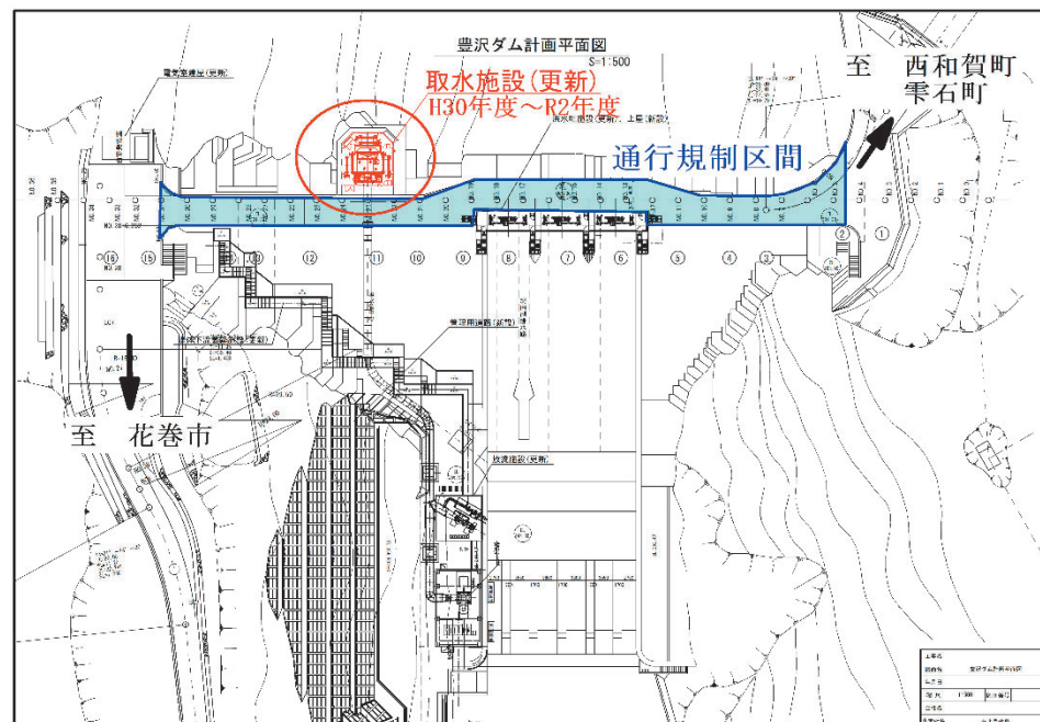
<豊沢ダム計画平面図>
